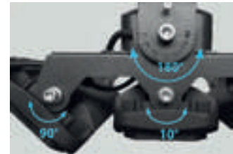
Schwenkbare Lichtbündel
